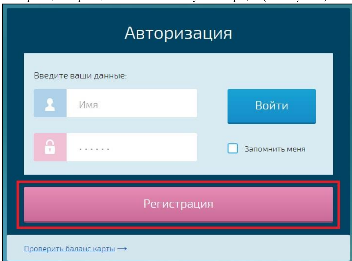
Рисунок 2 — страница авторизации.
