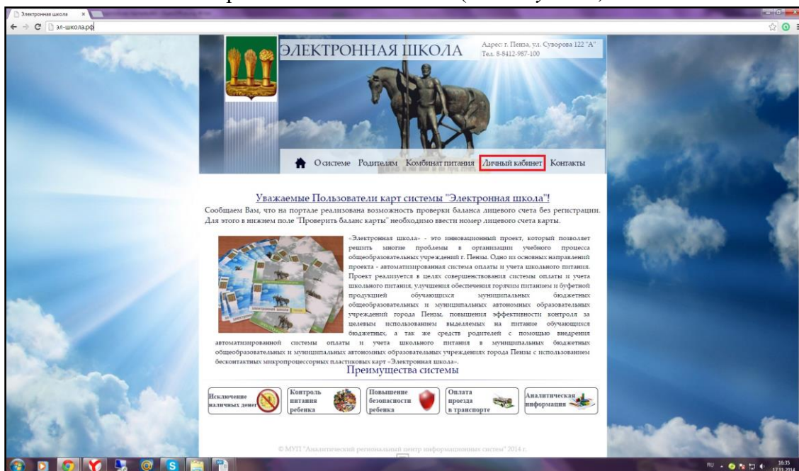
Рисунок 1 — личный кабинет.
